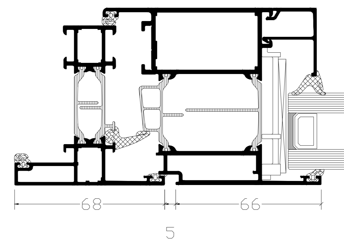
STANDAARD VLEUGEL
