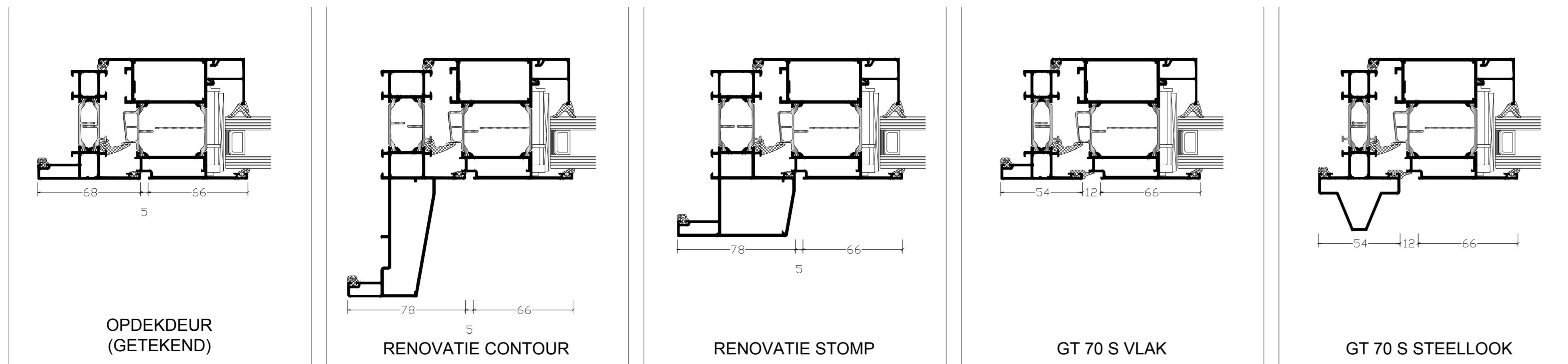
RENOVATIE CONTOUR
