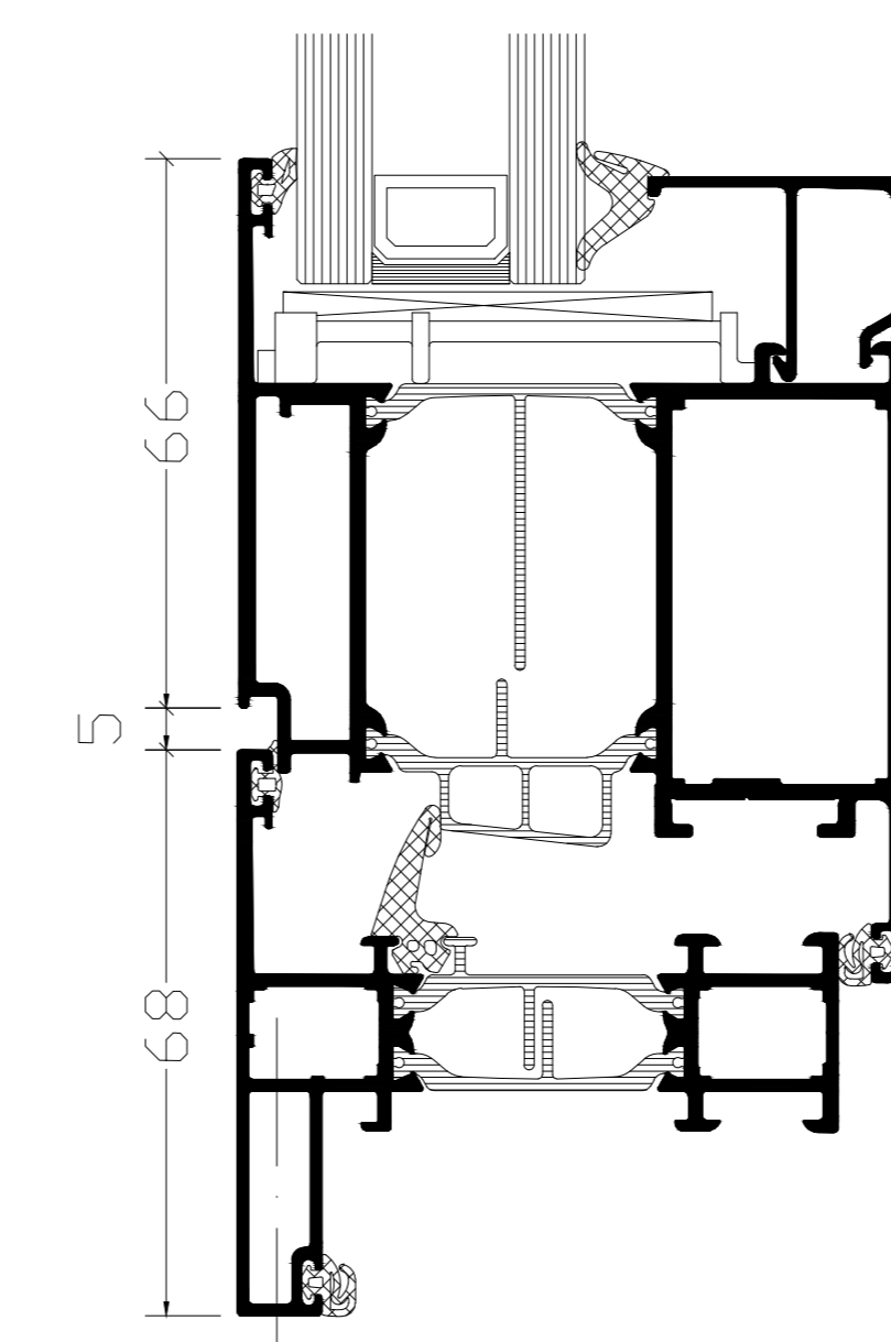
VERBORGEN WATERAFVOER
