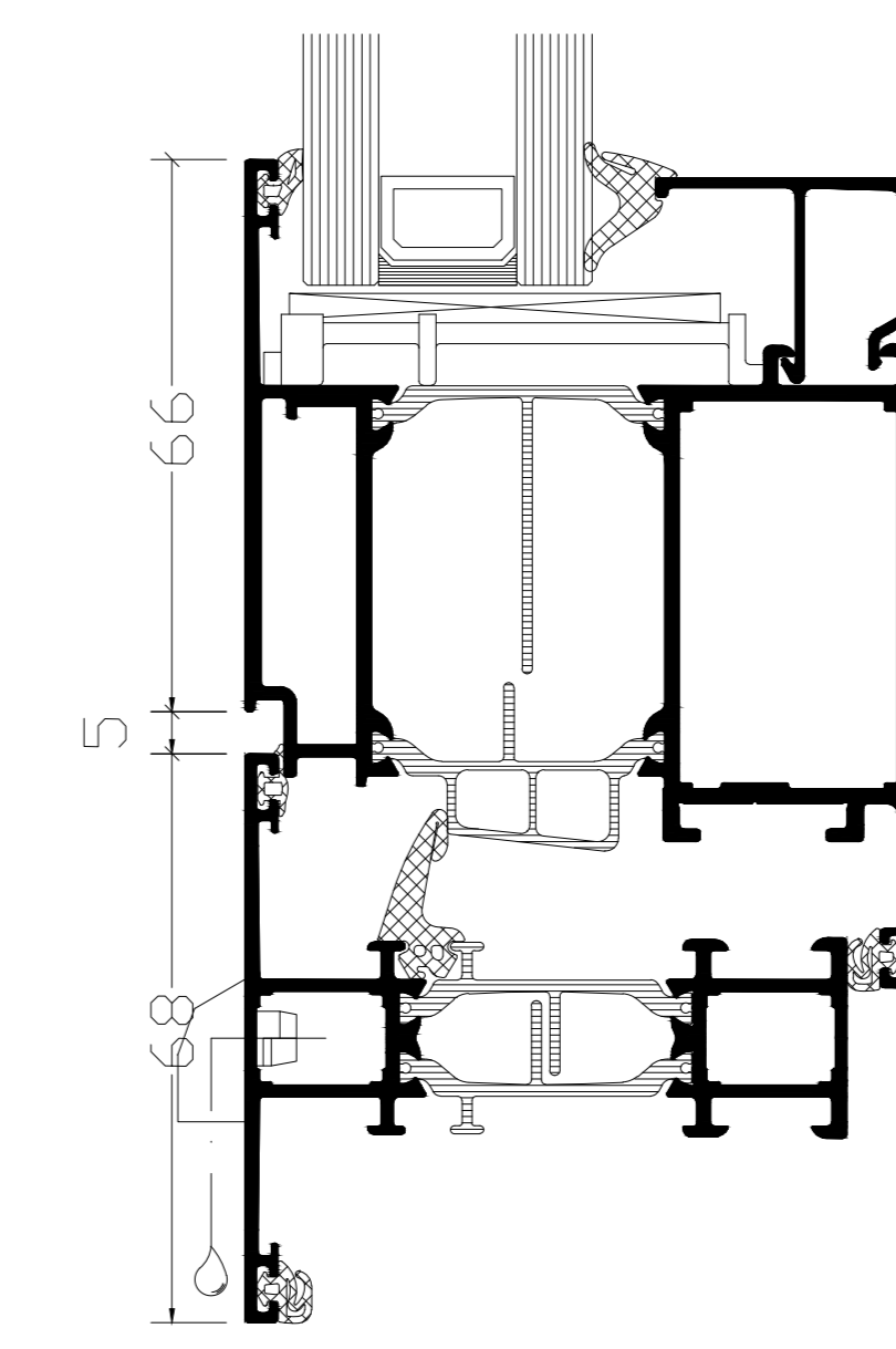
GECOMPARTIMENTEERDE WATERAFVOER
