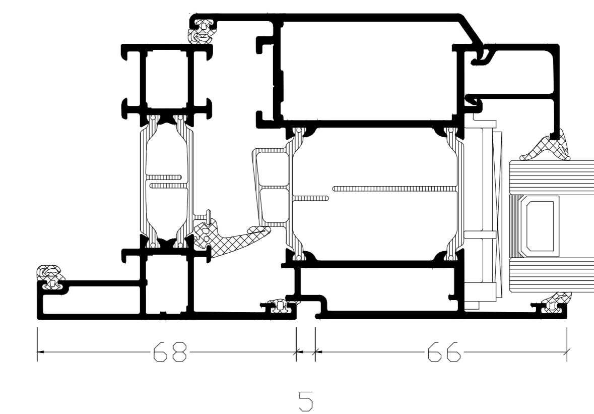
SOFTLINE VLEUGEL
