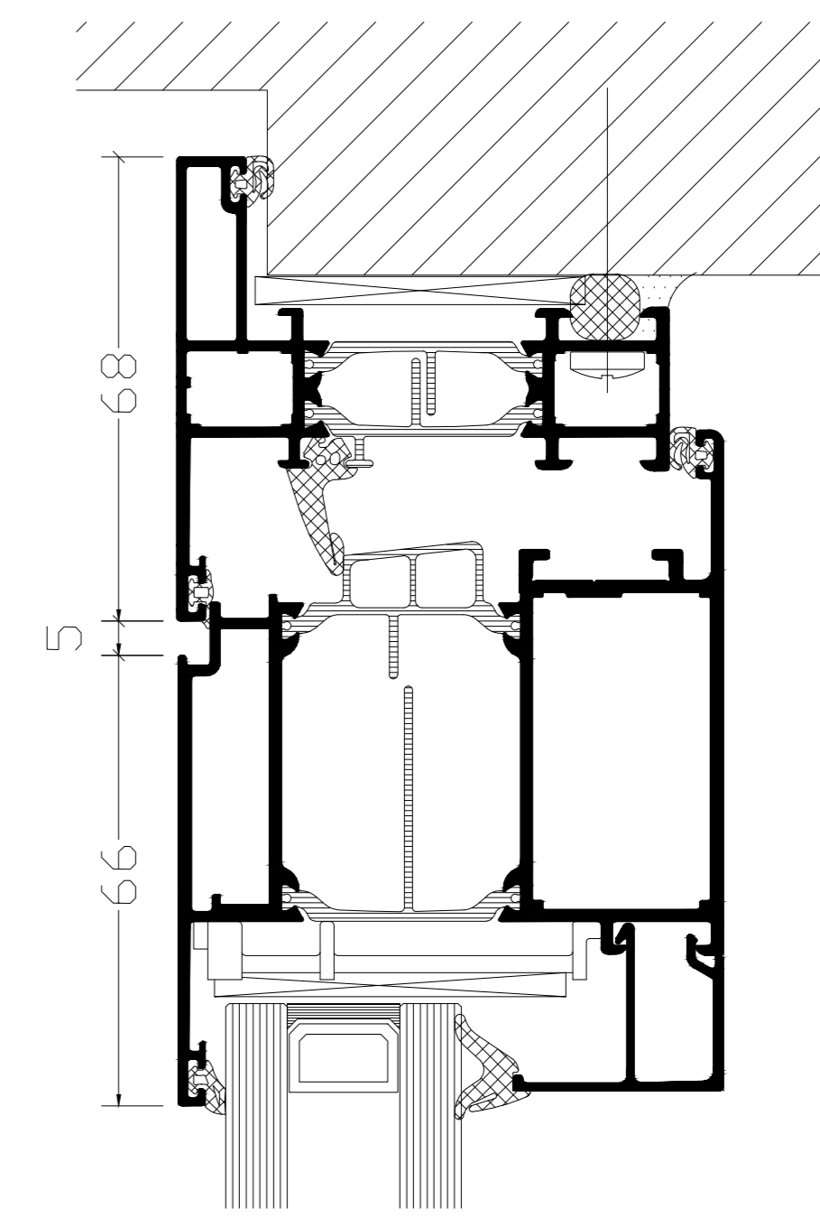
AANSLUITING BOVEN
