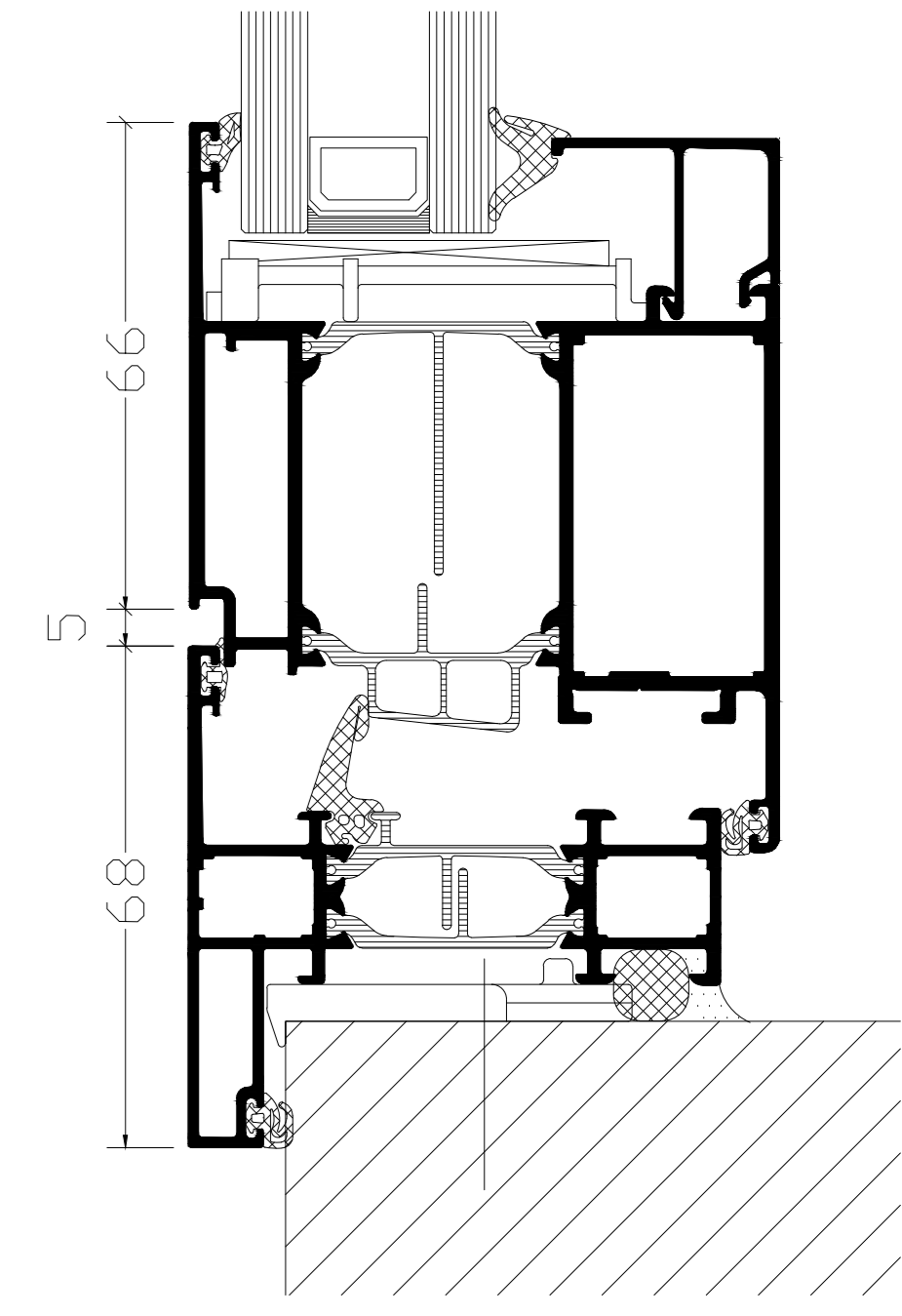
AANSLUITING ONDER
