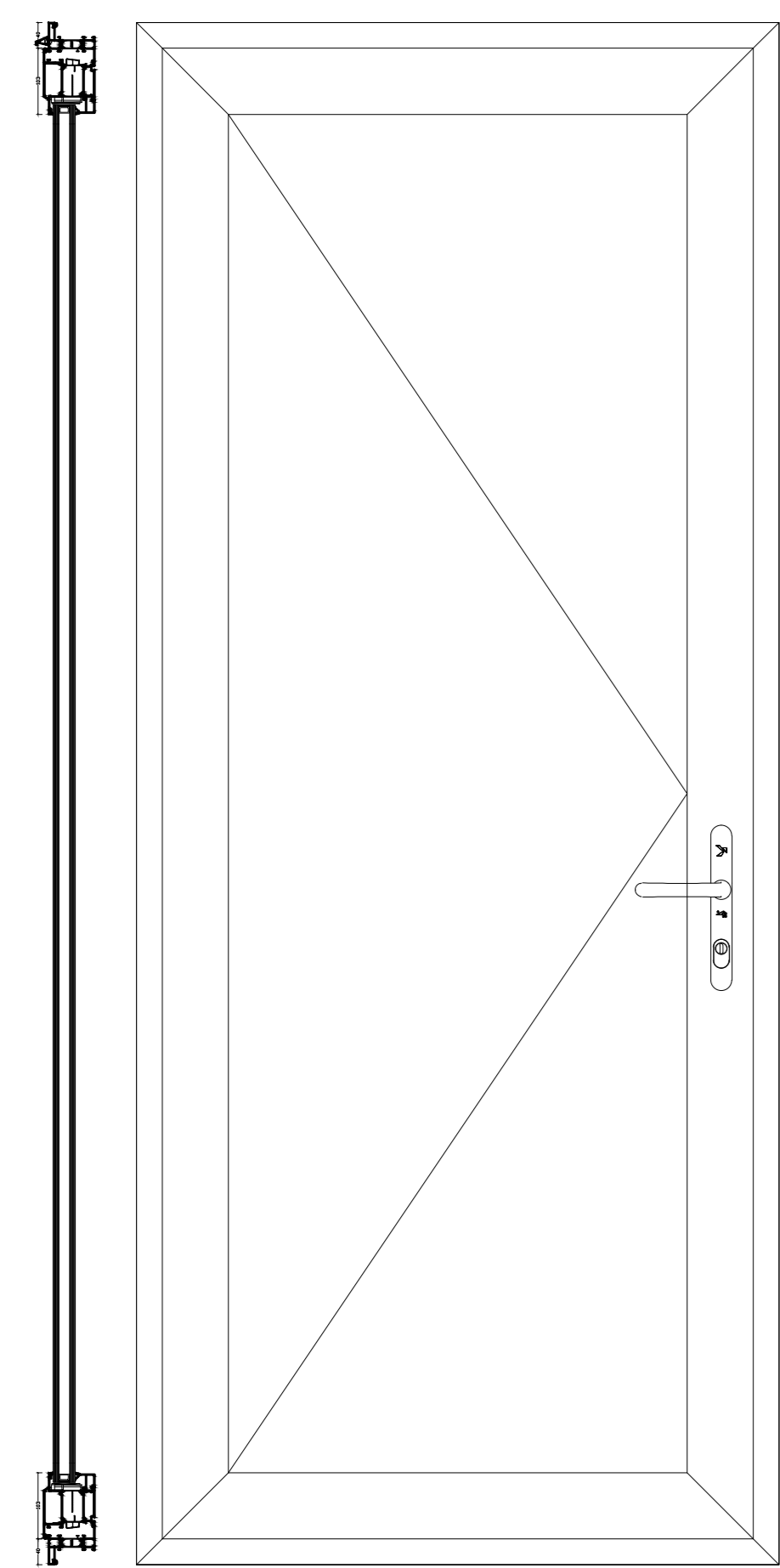
OPDEKDEUR BUITENDRAAIEND
