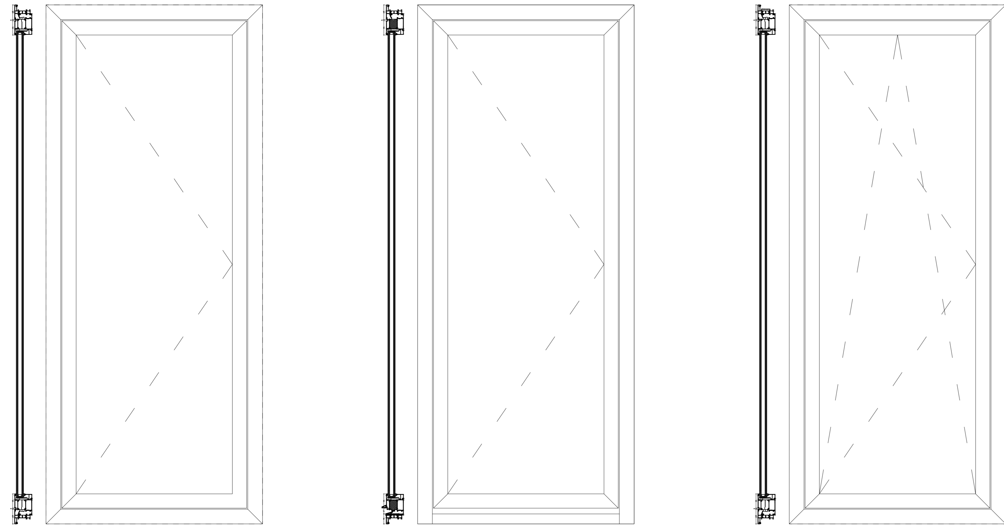
OPDEKDEUR BINNENDRAAIEND
